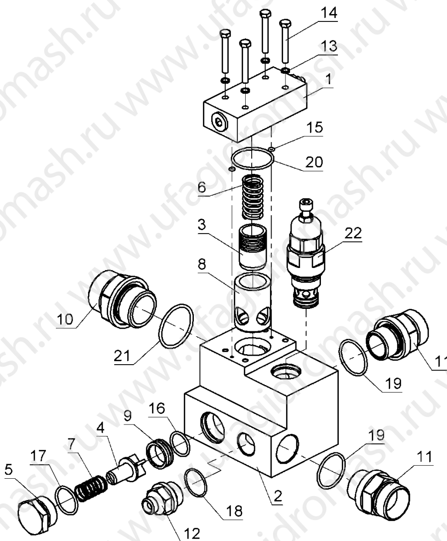
Блок клапанов ГСЭ.003.00
