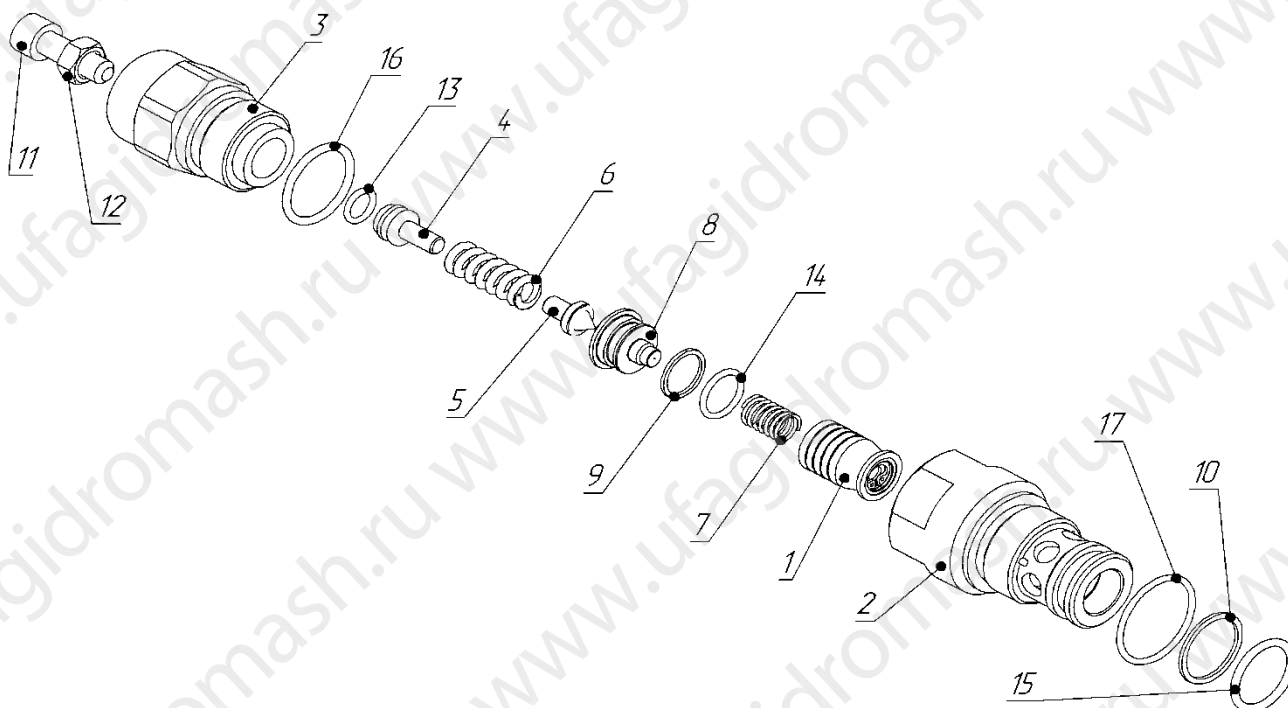
Клапан предохранительный VMP 20
