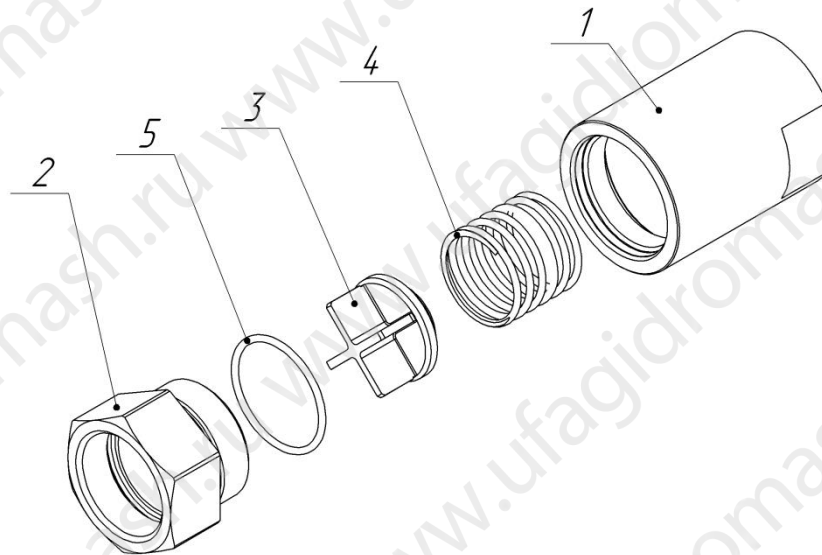
Клапан ГСЭ.021.00
