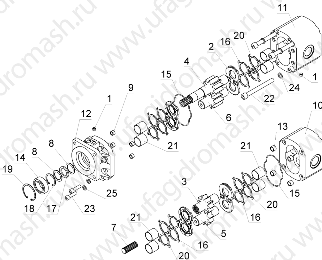
Гидромотор ГМ40.109.087
