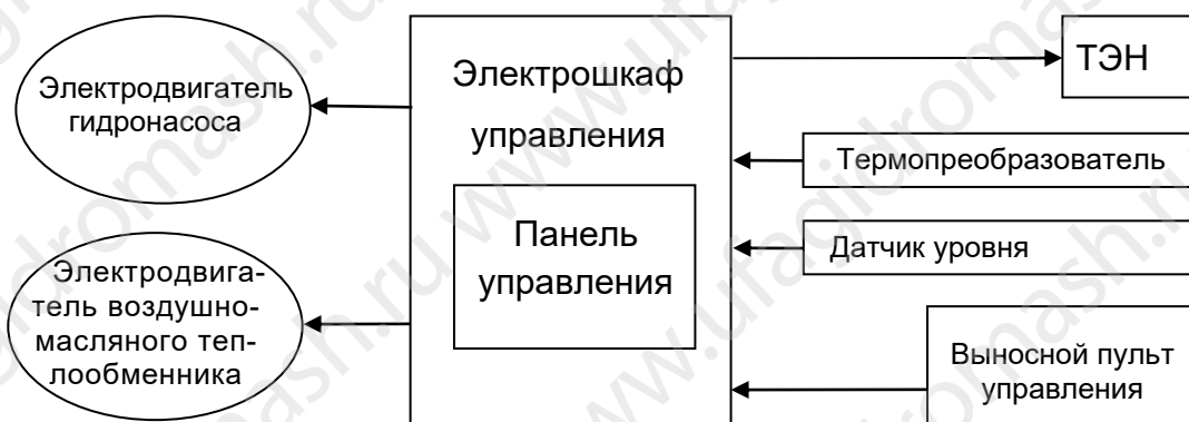
Рисунок 2 Структурная схема
