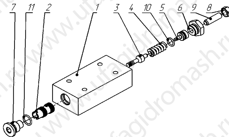
Клапан отсечки ГСЭ.004.00
