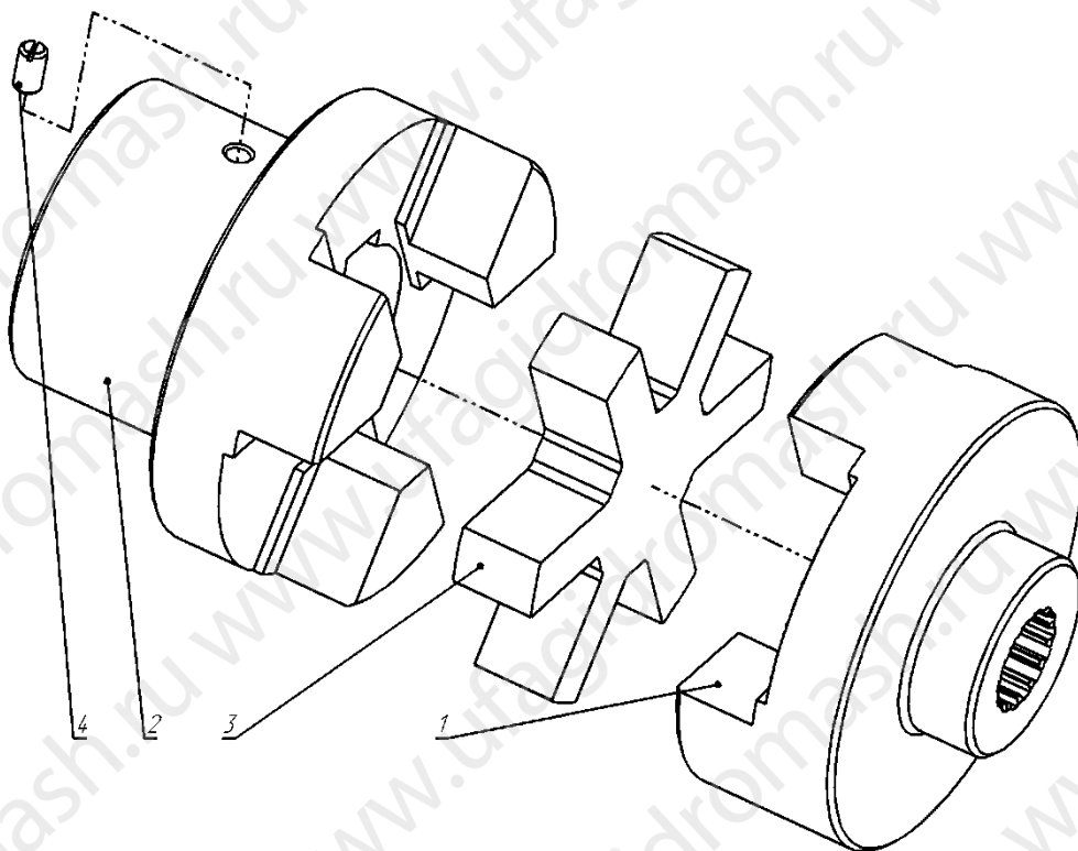
Рисунок 9 Муфта ГСЭ.505.00-01
