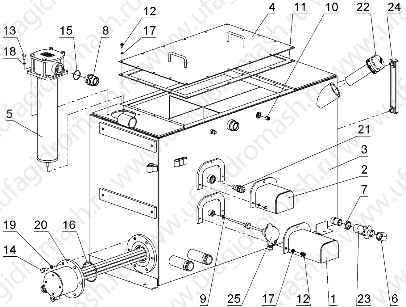
Бак в сборе ГСЭ.110.00
