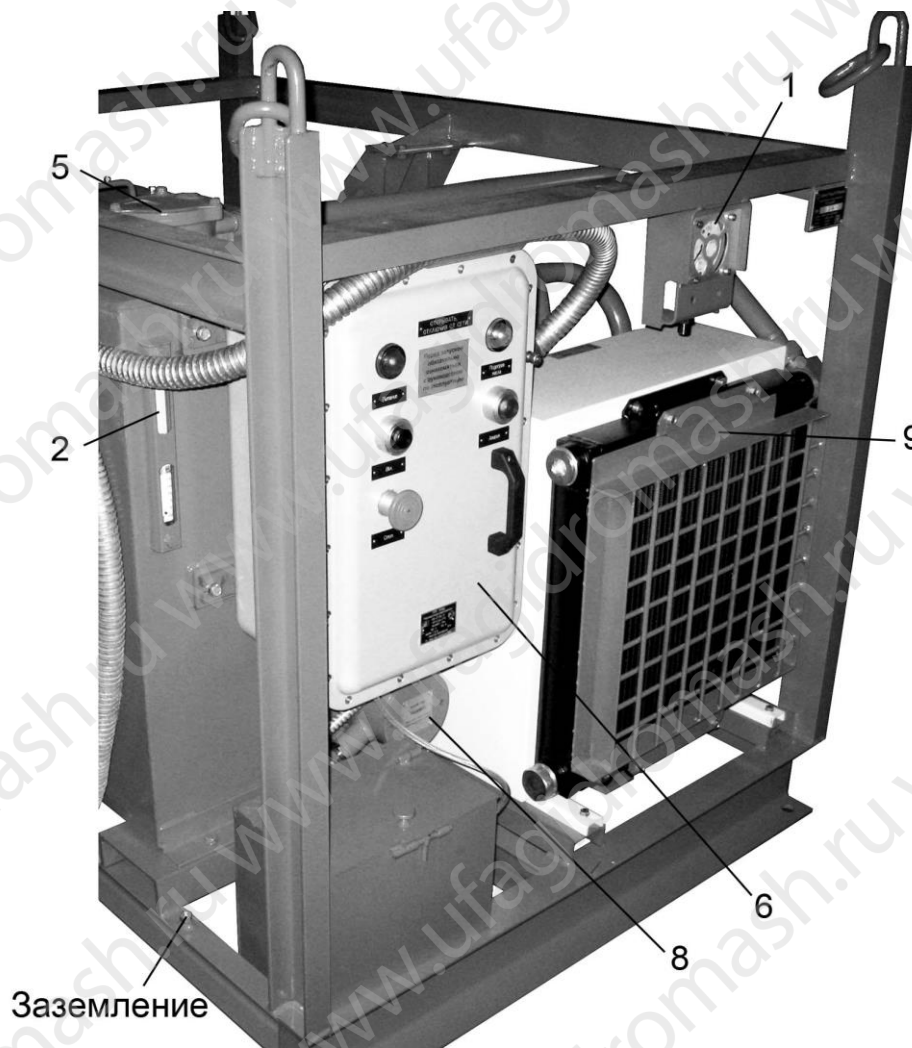
Рисунок 1 Гидростанция
