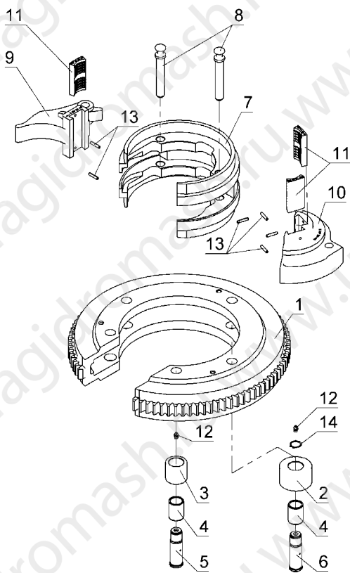
Рисунок 16 Ротор в сборе ГК32.042.000
