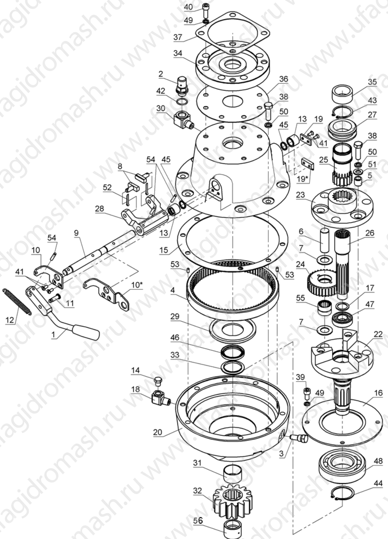
Рисунок 15 Коробка передач
