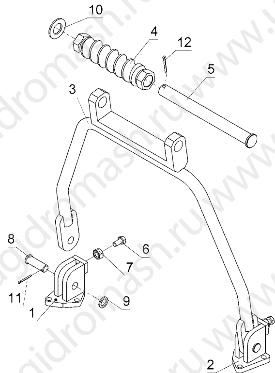
Рисунок 17 Подвеска в сборе
