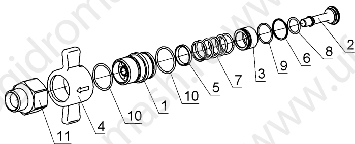
Ниппель БРС.32.02.000-01
