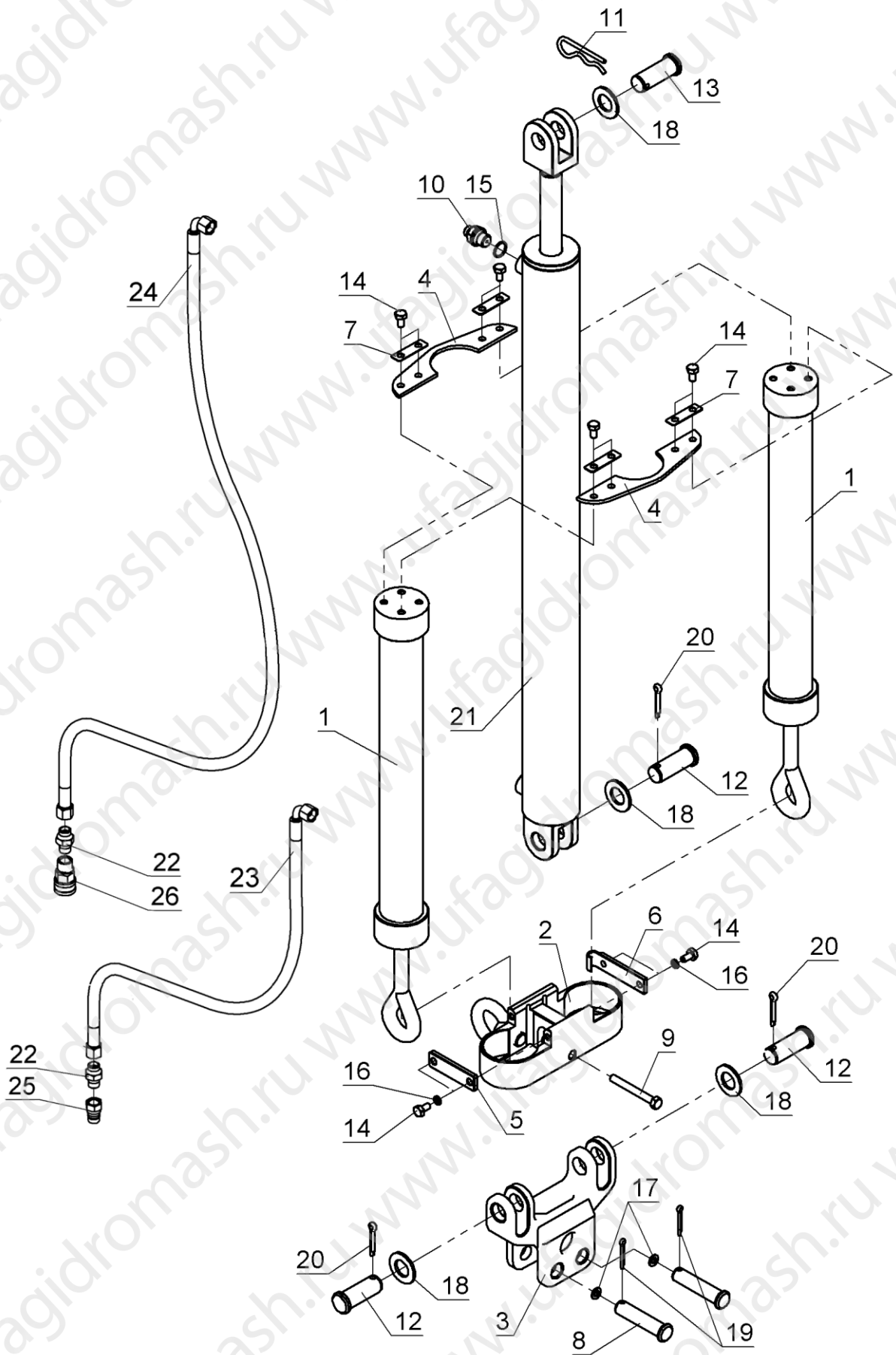
Рисунок 20 Цилиндр подвески в сборе
