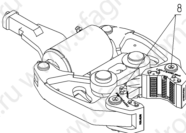
Схема смазки устройства гидравлического стопорного
