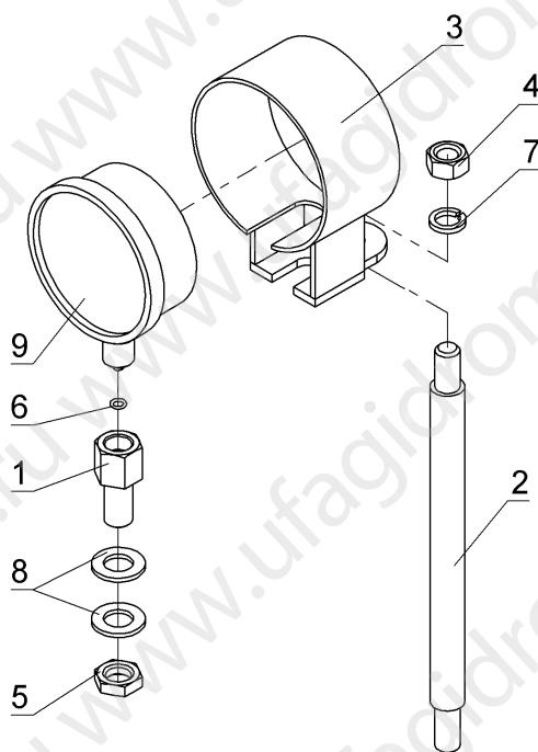
Рисунок 22 Манометр
