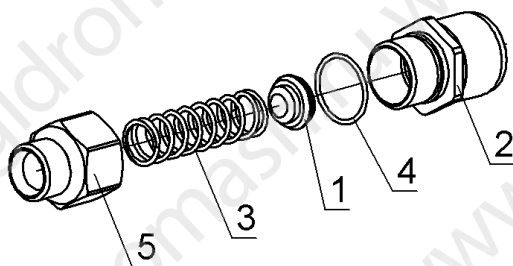
Муфта БРС.01.000-01
