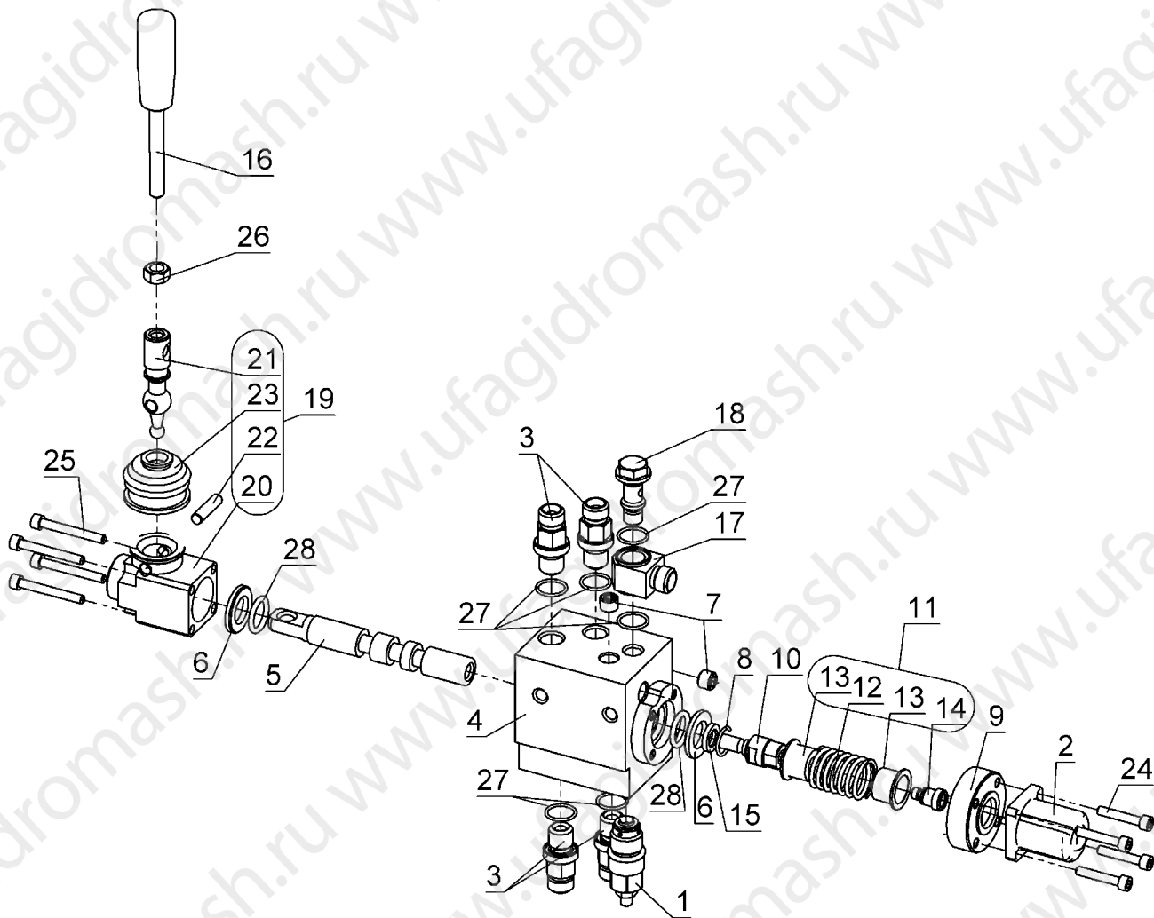
Рисунок 32 Модуль гидравлический стопорного устройства ГК18.240.000
