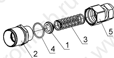
Муфта БРС.32.01.000
