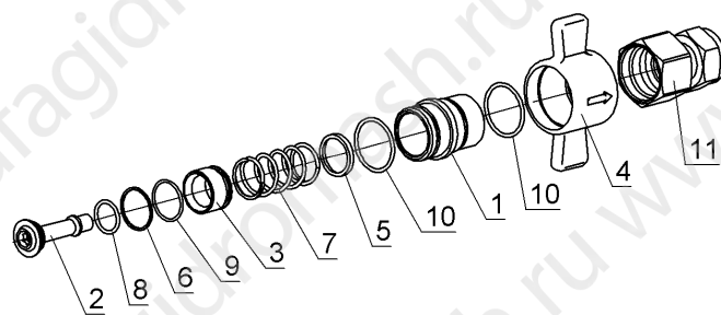
Ниппель БРС.02.000
