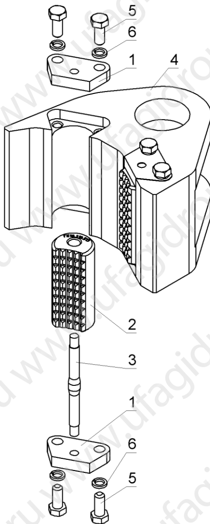
Рисунок 31 Челюсть в сборе ГК32.410.510
