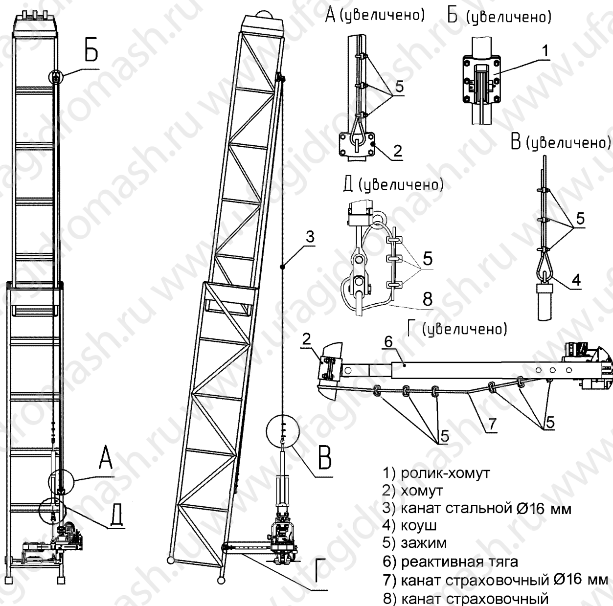
Рисунок 3 Рекомендуемая схема монтажа гидроключа
